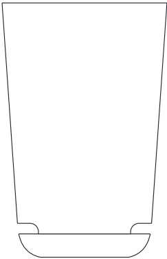
DUETTO GRANDE Ø 39 cm e h 58 cm, Ø 31 cm e h 5,5 cm (sottovaso)
